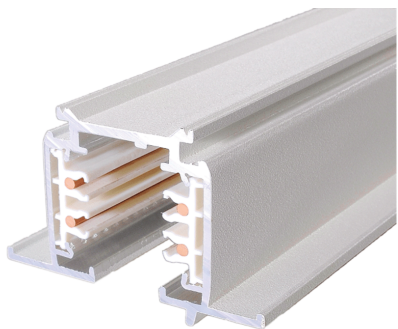
參數表 | 四線三迴路嵌入式導軌-2米 (2000mm)
